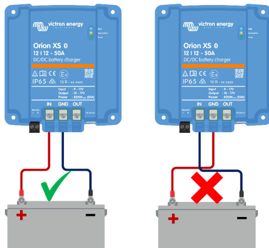
Esempio di polarità corretta ed erronea (inversa) della batteria
