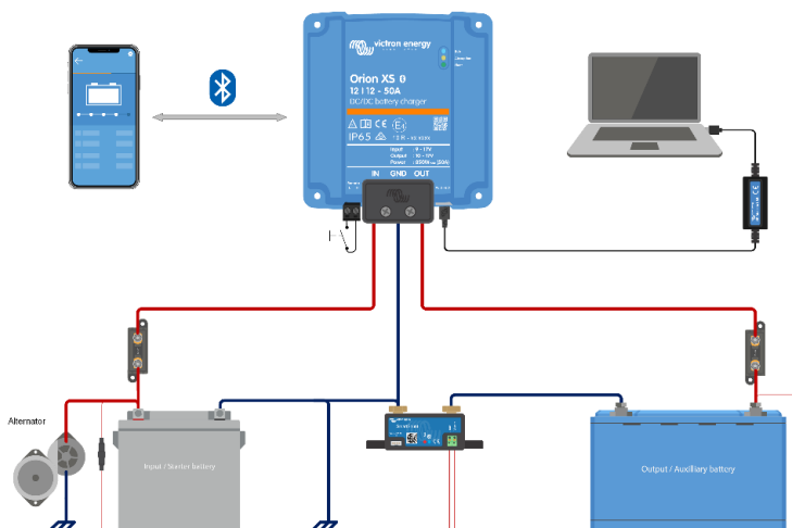
Impostazione tipica del collegamento come caricabatterie CC-CC
