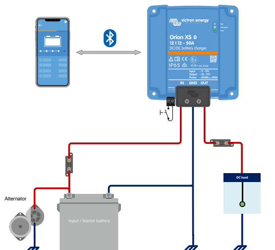
Impostazione tipica del collegamento come alimentatore CC-CC
