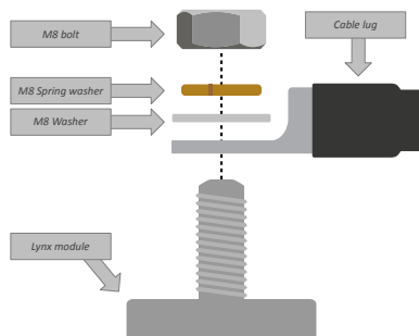
Figura 4. Corretta sequenza di montaggio dei cavi CC
