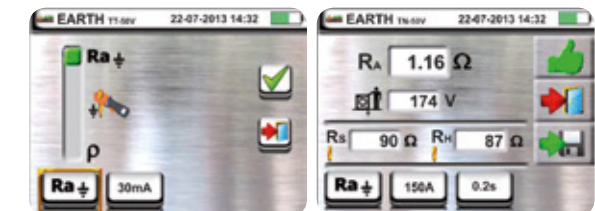
Misura di resistenza di terra con metodo Voltamperometrico.
