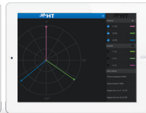
Diagramma vettoriale delle tensioni e correnti.
