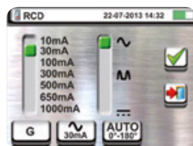
Selezione tipo e corrente di intervento RCD
