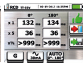
Risultati test AUTO su RCD
