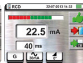
Risultato test a rampa su RCD
