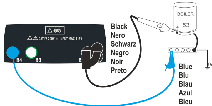
Fig. 11: Prova di continuità tramite puntale remoto
