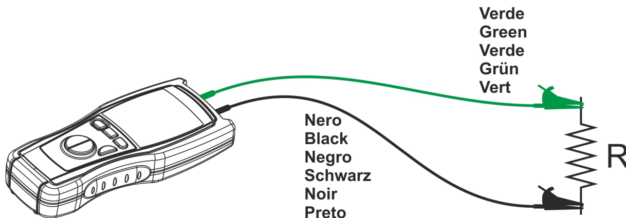
Fig. 5: Connessione dei terminali dello strumento
