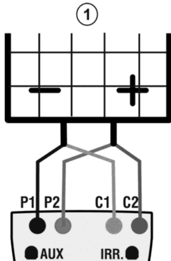
Fig. 13: Coll. strumento al modulo/stringa FV per prove IVCK senza misura mis. Irragg.
