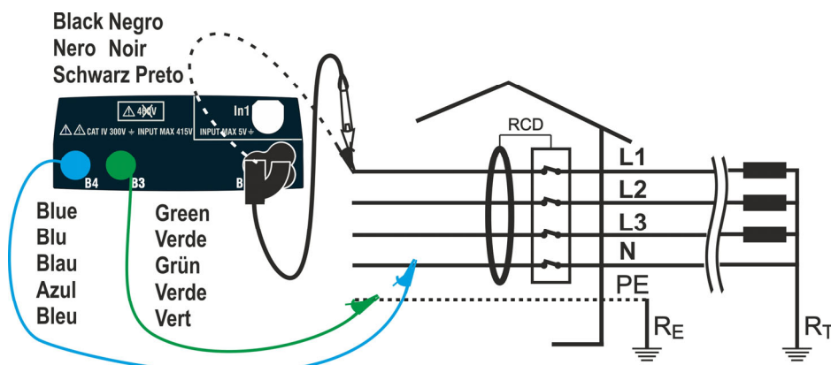
Fig. 21: Collegamento per sistema Trifase L1-L2-L3-N tramite cavi singoli e puntale
