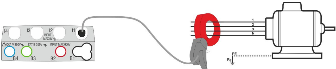
Fig. 25: Misurazione indiretta della corrente di dispersione in impianti trifase
