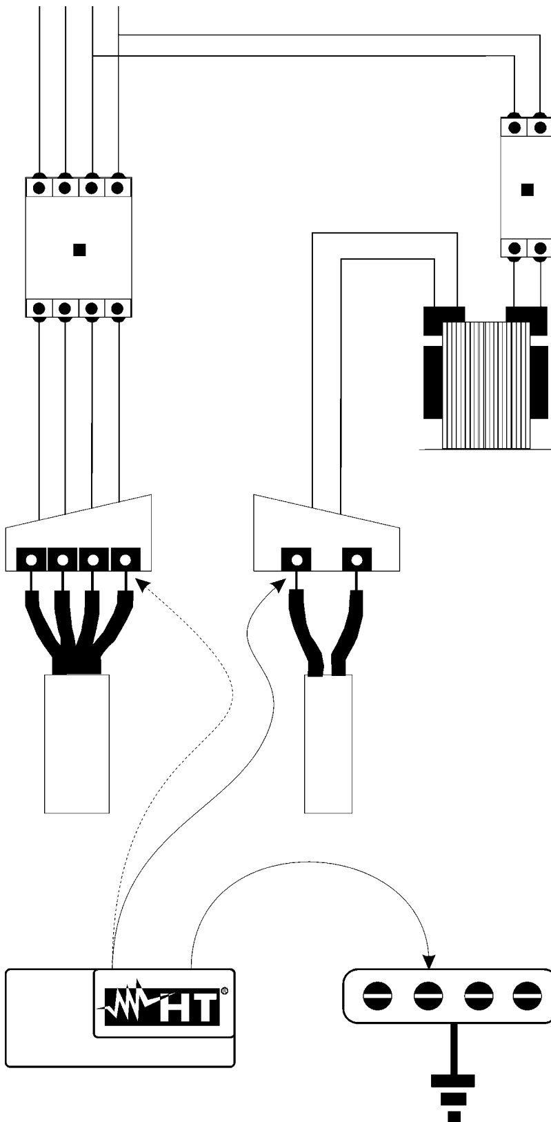
Fig. 51: Misure di separazione tra circuiti in un impianto
