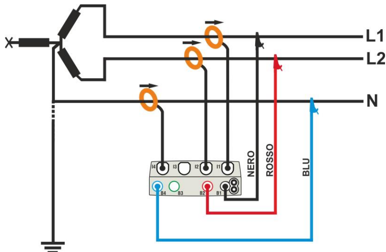
Fig. 43: Collegamento per misura su impianto Bifase 3\phi -2EI. \frac{1}{2} – sistemi USA
