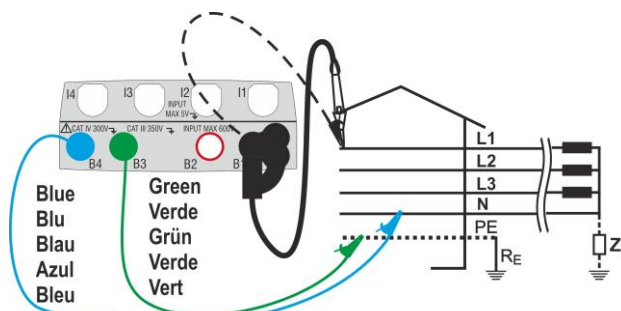
Fig. 22: Misura L-PE in sistemi IT con cavi singoli e puntale remoto
