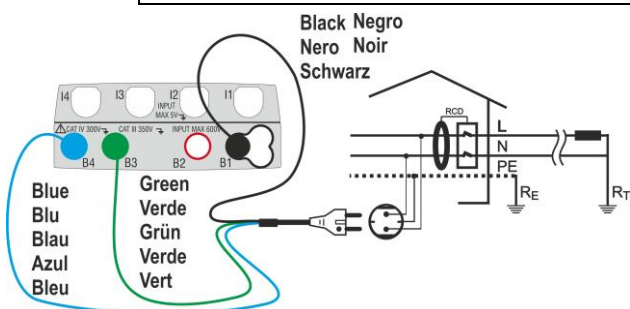
Fig. 10: Collegamento in sistema monofase tramite spina shuko
