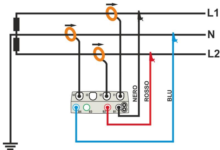
Fig. 44: Collegamento per misura su impianto Bifase 1\phi -PresaCentrale – sistemi USA
