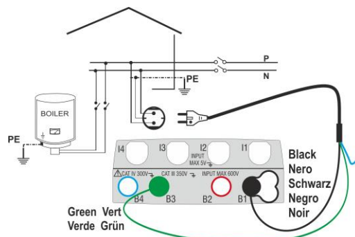
Fig. 9: Verifica dell'isolamento tramite spina shuko
