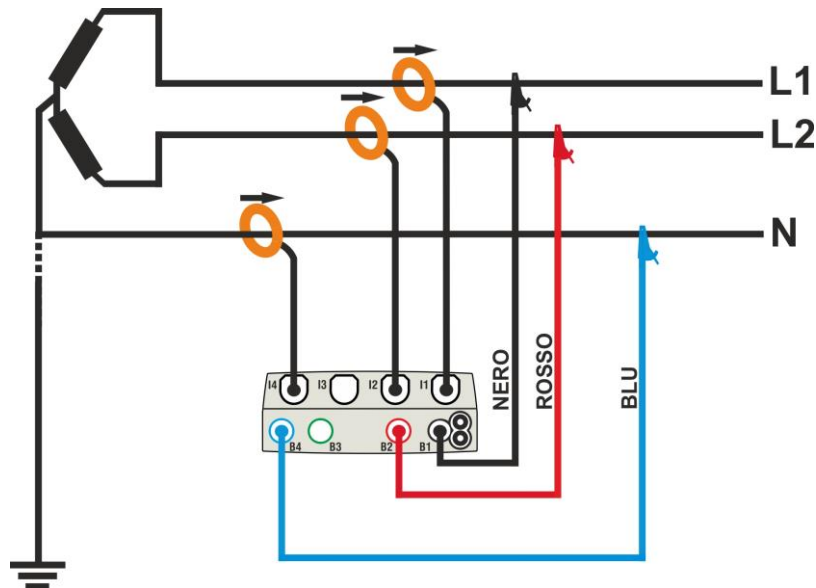
Fig. 42: Collegamento per misura su impianto Bifase 3\phi -Y Aperta – sistemi USA
