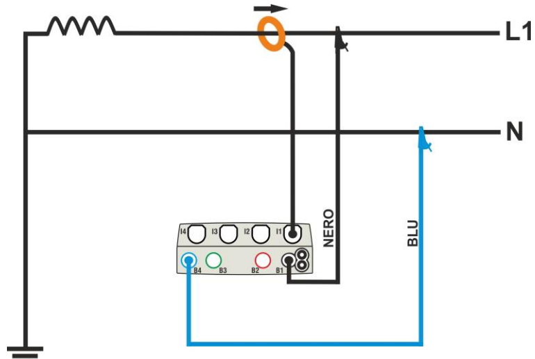
Fig. 36: Collegamento per misura su impianto Monofase 1\phi -2FILI
