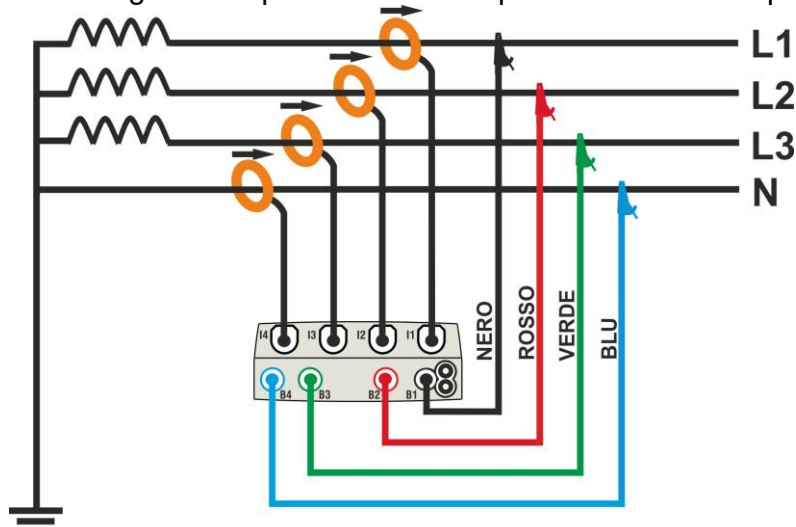
Fig. 37: Collegamento per misura su impianto Trifase 3\phi -4FILI
