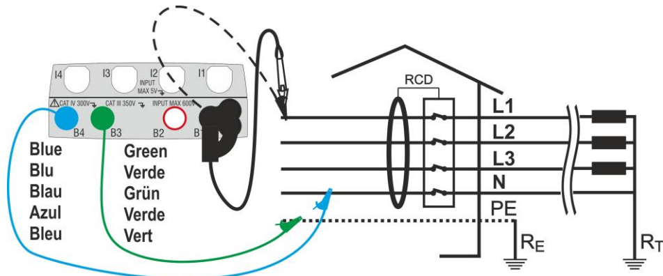
Fig. 13: Collegamento in sistema trifase con cavi singoli e puntale remoto
