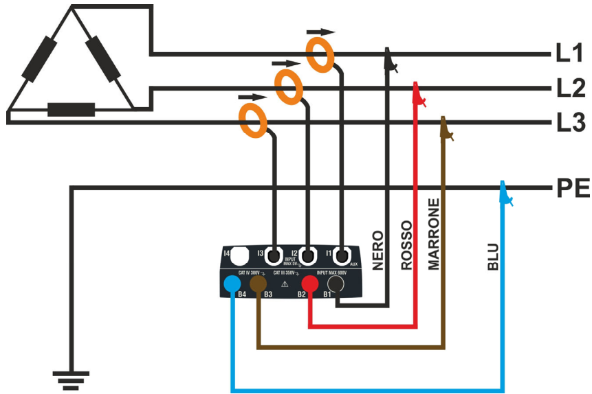
Fig. 12: Collegamento per misura su impianto Trifase 3\phi -ARON
