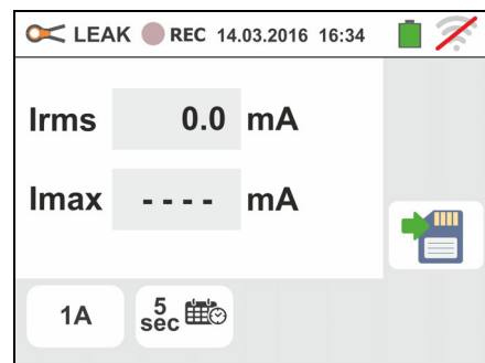
Fig. 7: Misurazione diretta della corrente di dispersione in impianti trifase
