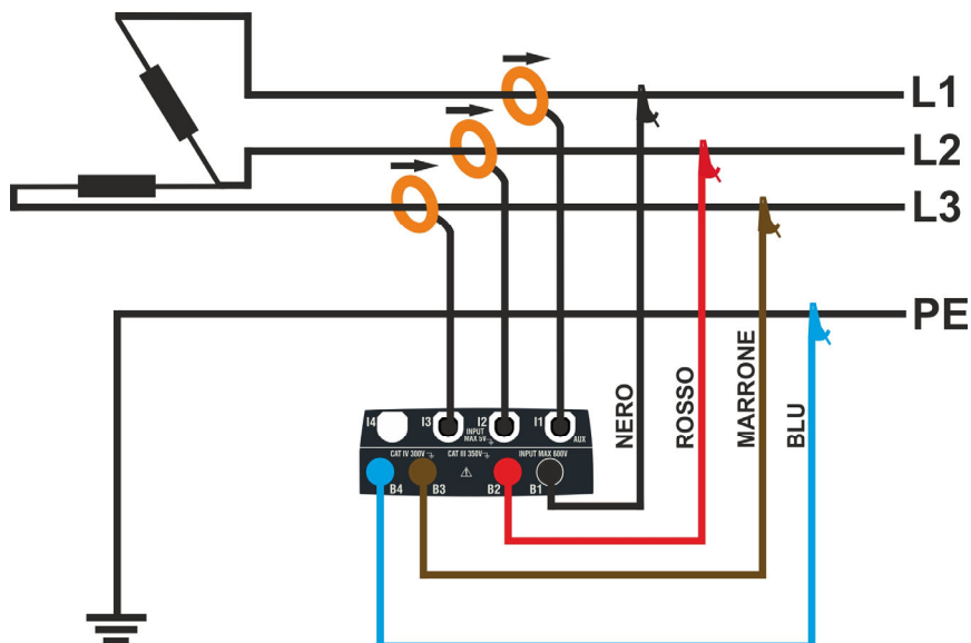
Fig. 14: Collegamento per misura su impianto Trifase 3\phi - \Delta Aperto – sistemi USA
