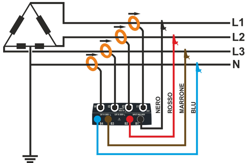
Fig. 13: Collegamento per misura su impianto Trifase 3\phi -High Leg – sistemi USA
