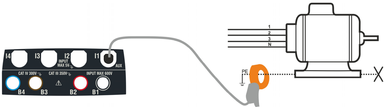
Fig. 7: Misurazione diretta della corrente di dispersione in impianti trifase
