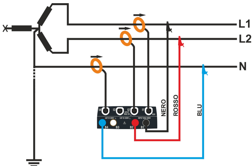
Fig. 16: Collegamento per misura su impianto Bifase 3\phi -2EI. \frac{1}{2} – sistemi USA
